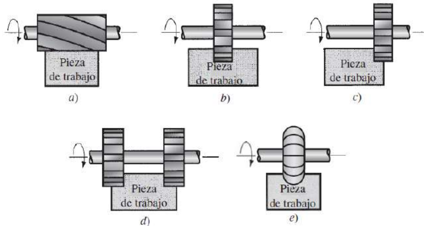
Figura 4. Fresado periférico: a) fresado de bloque, b) ranurado, c) fresado lateral, d) fresado paralelo simultáneo y e) fresado de forma[1].
